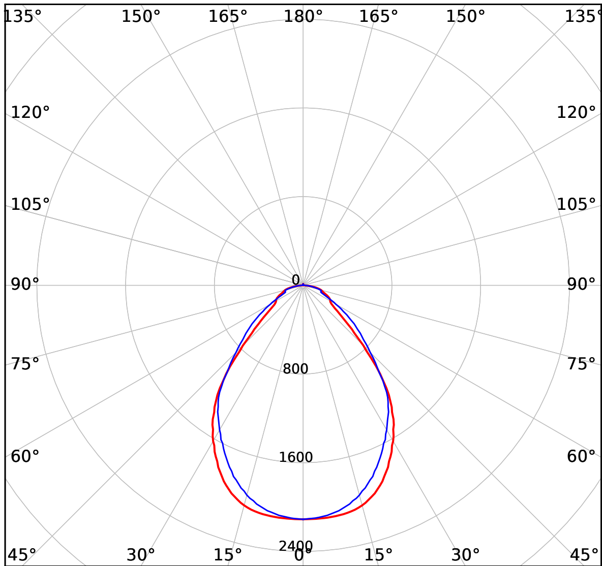
cd 3900 lm — C0-C180 — C90-C270
