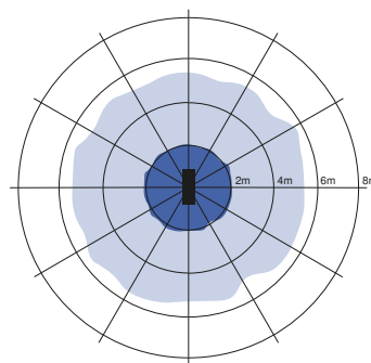
Installation - Deckenmontage Empfohlene Montagehöhe 2.5-4m
